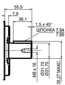
Код вала W
